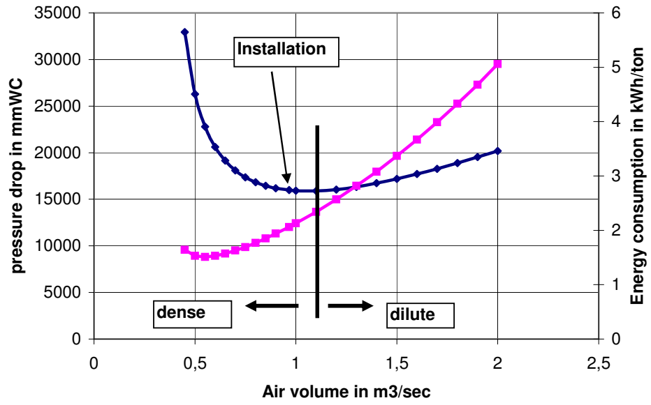
Zenz diagram
